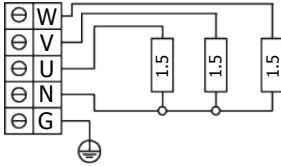
ARI3-45NS-WL 4,5 kW
